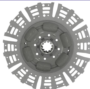
DUPLO EXTERNO MB 2638 10 ESTRIAS 400MM (SACHS 5576)
