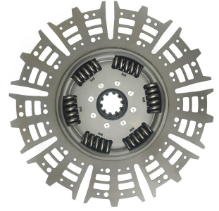
VW / MB / IVECO 10 ESTRIAS 6 MOLAS ABERTAS 430MM
