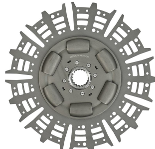
MB1938 AXOR 18 ESTRIAS 430MM (SACHS 5535)
