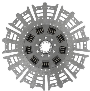
VOLVO NL12 9 MOLAS 10 ESTRIAS 430MM
