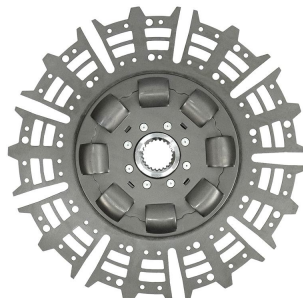
SCANIA 113 8 MOLAS 22 ESTRIAS 430MM
