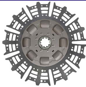
SCANIA / MERCEDES O-400 10 ESTRIAS 8 MOLAS 430MM (SACHS 5705)
