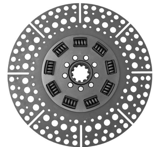
MB 1620 SACHS 9 MOLAS 350MM
