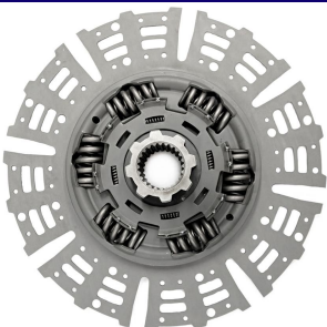
DUPLO EXTERNO VOLVO FH 24 ESTRIAS 400MM (SACHS 5583)
