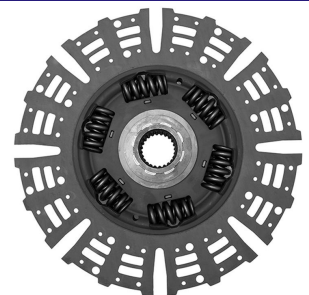
DUPLO INTERNO VOLVO FH 24 ESTRIAS 400MM (SACHS 5577)
