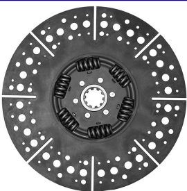
VW CONSTELLATION 10 ESTRIAS C/ PRÉ DAMPER 395MM (SACHS 5597)
