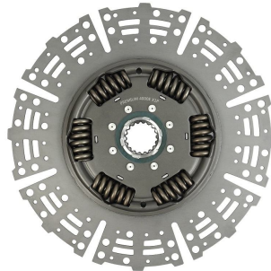
EXTERNO NEW ACTROS 400MM (SACHS 5582)
