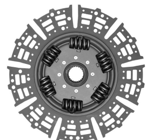
MB / SCANIA SÉRIE 5 / VOLVO 24 ESTRIAS PRÉ-AMORTECIMENTO 430MM (SACHS 5453)
