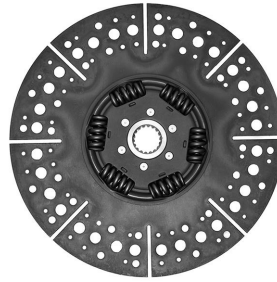
MB 1722 18 ESTRIAS C/ PRÉ-DAMPER 4 MOLAS 395MM (SACHS 5766)
