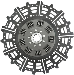
SCANIA 110/111 ESTRIA GROSSA 10 ESTRIAS 420MM (SACHS 5331)
