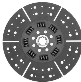
MB 1313 310MM (SACHS 5391)
