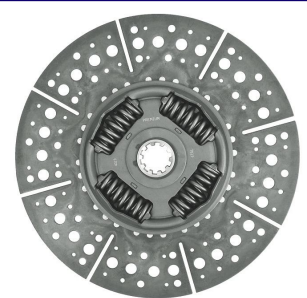
MOTOR MAN 10 ESTRIAS 4 MOLAS 395MM
