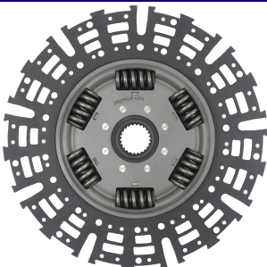
VOLVO D-13 / I-SHIFT 24 ESTRIAS 430MM (SACHS 5012)
